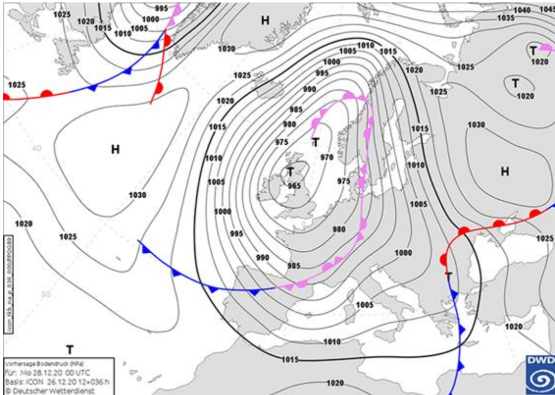
Slika 1. Prognoza prizemnog tlaka zraka modela DWD i frontalni poremećaji u ponedjeljak, 28. 12. u 00 UTC
