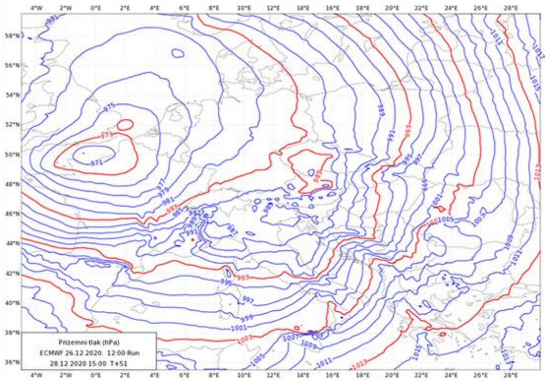
Slika 2. Prognoza prizemnog tlaka zraka modela ECMWF za ponedjeljak 28. 12. u 15 UTC
