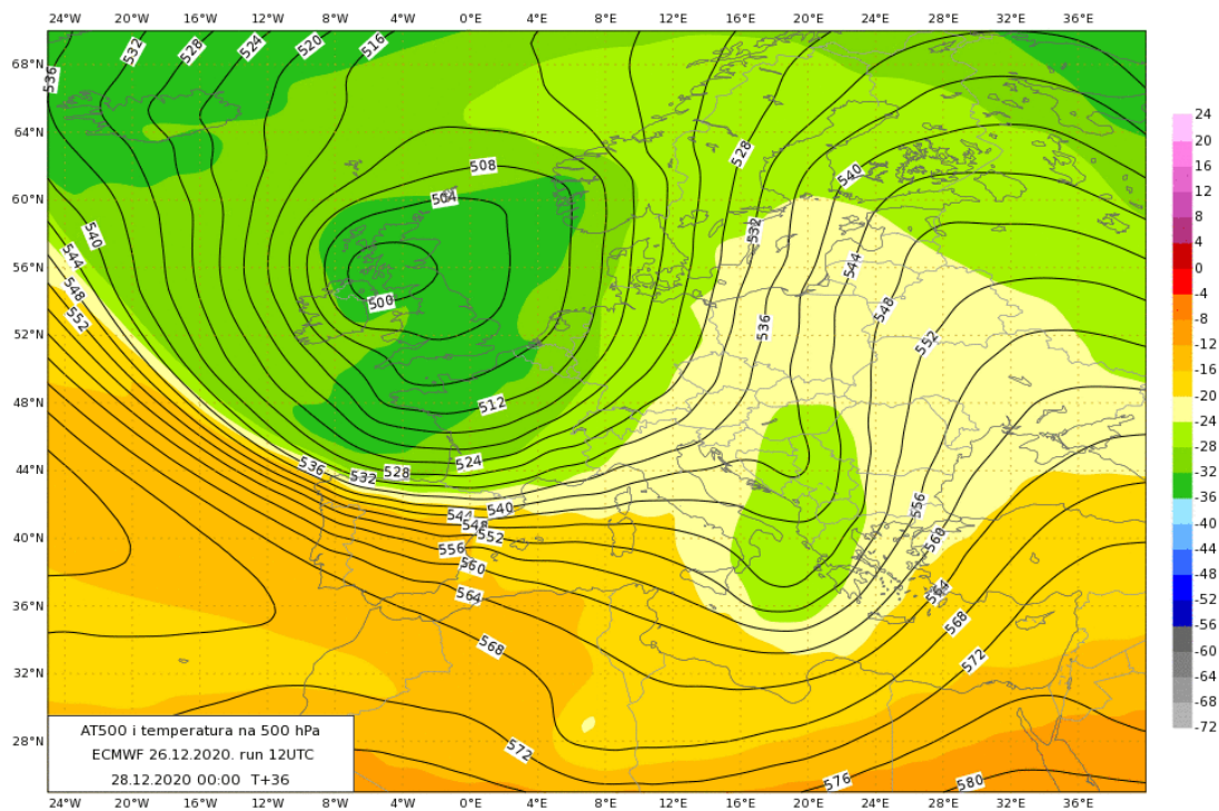
Slika 4. Duboka termobarička dolina i visinska ciklona. ECMWF prognoza temperature i geopotencijala na 500 hPa plohi od 28. 12. u 00 UTC do 01. 01. 2021. u 00 UTC.
